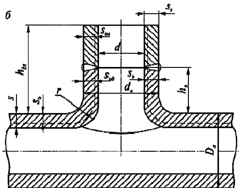
Рис.4.3. Тройник: а - сварной; б - штампованный
