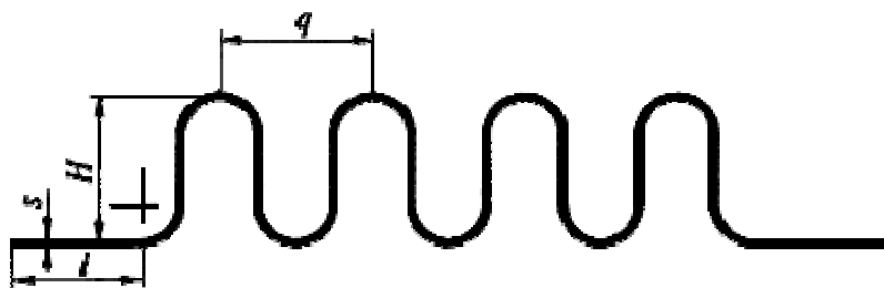
Рис.5.5. Гибкий элемент компенсатора
